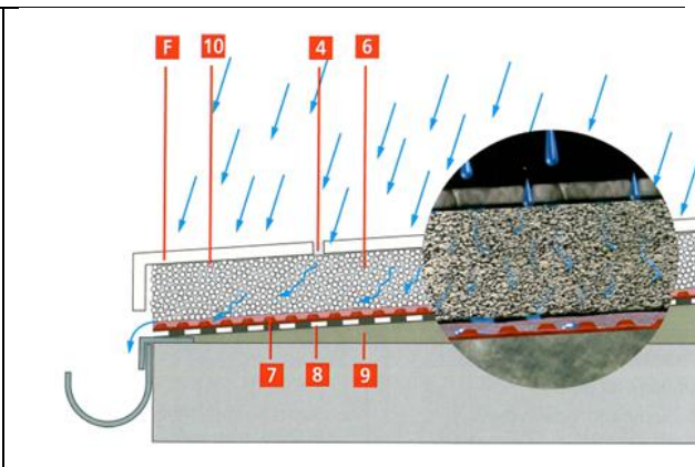
Figur 7: Materialsammensetning av drenerende mørtler og matter
